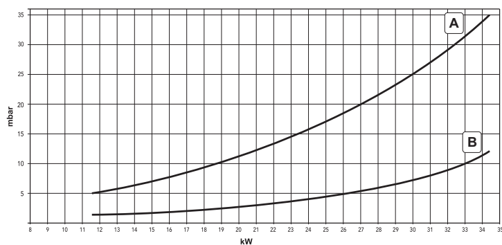
fig. 34 - DIVAtop 60 F 32
