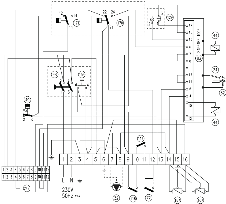
мал. 12 - Електрична схема підключення мод. 119 - 136
