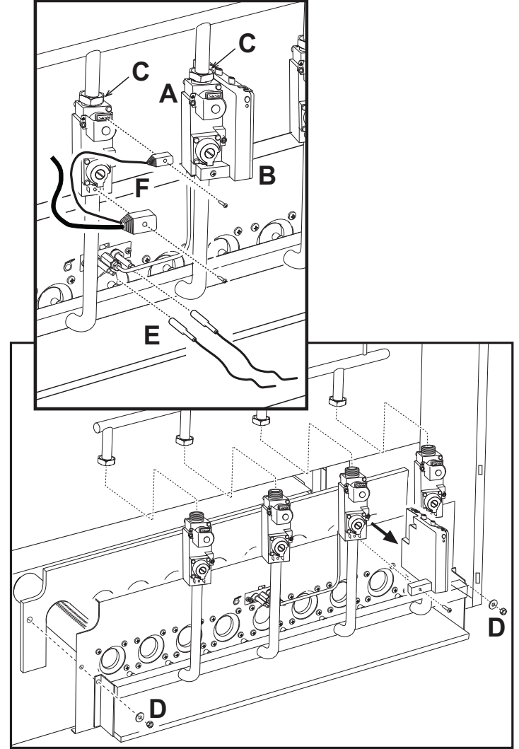
şek. 7 Brülörlerin sökülmesi ve temizlenmesi
