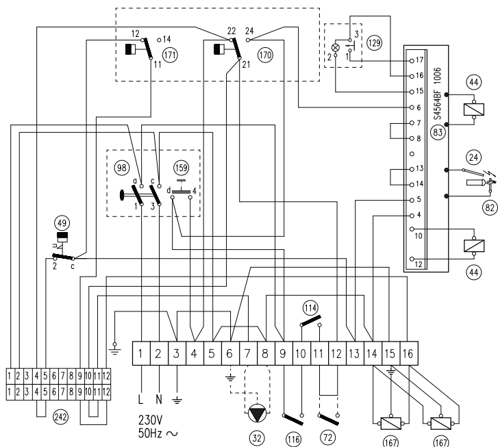
fig. 12 - Esquema eléctrico de conexión mod. 119 - 136
