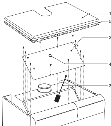
fig. 9 - Limpieza de la caldera
