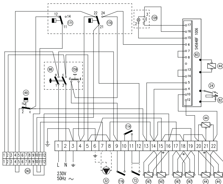
fig. 14 - Esquema eléctrico de conexión mod. 153 ÷ 289
