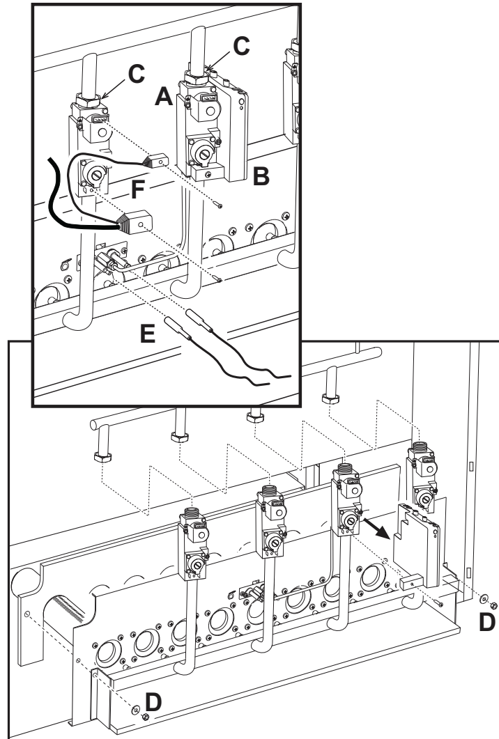
мал. 7 - Демонтаж та очищення вузлу пальників
