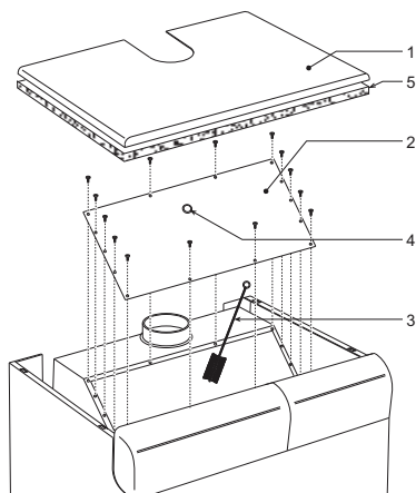
мал. 9 - Очищення котла
