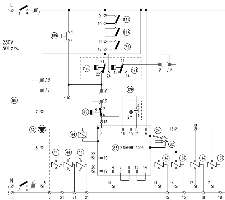
fig. 15 - Schema elettrico di principio mod. 153 ÷ 289
