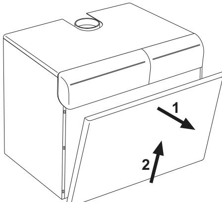
fig. 5 - Ouverture du panneau avant
