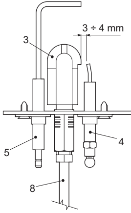
şek. 8 - Pilot brülör
