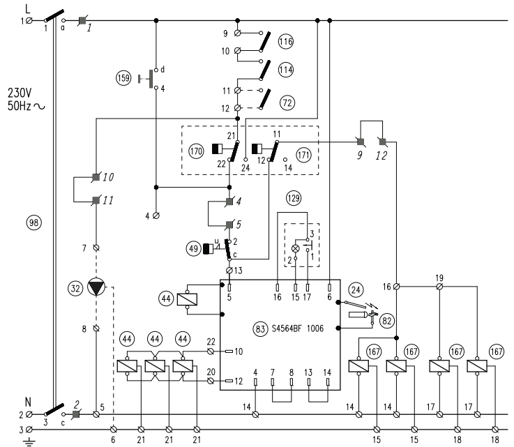
мал. 15 - Принципова електрична схема мод. 153 ч 289
