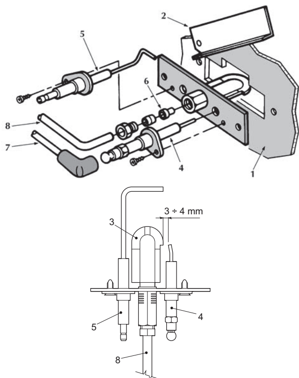
мал. 8 - Пілотний пальник
