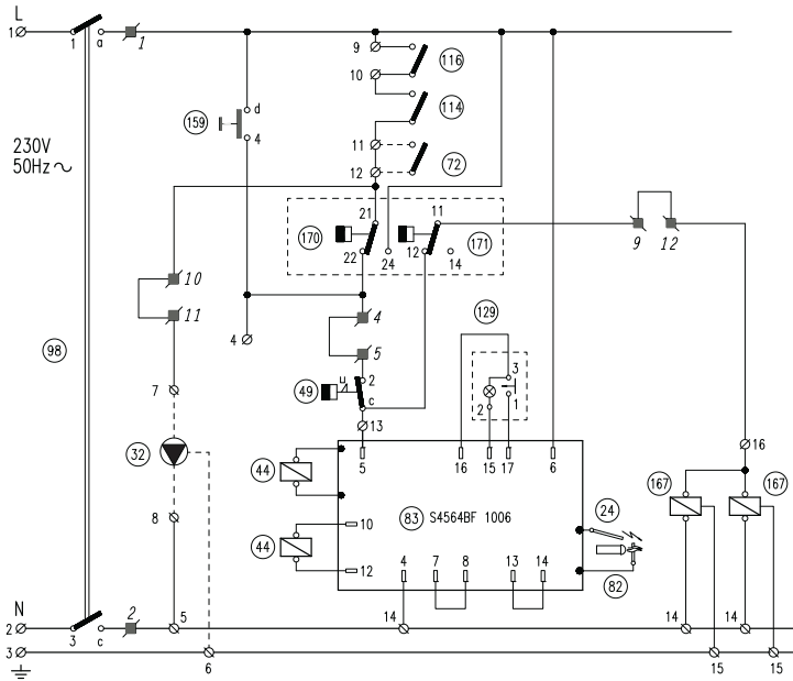
fig. 13 - Schéma électrique de base mod. 119 - 136
