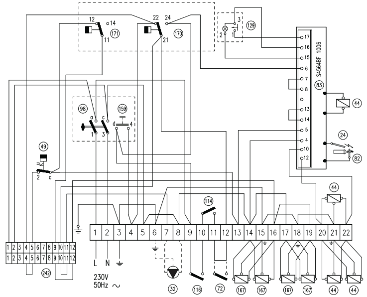
fig. 14 - Schéma électrique de raccordement mod. 153 + 289
