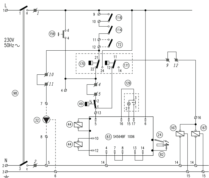
fig. 13 - Esquema eléctrico general mod. 119 - 136
