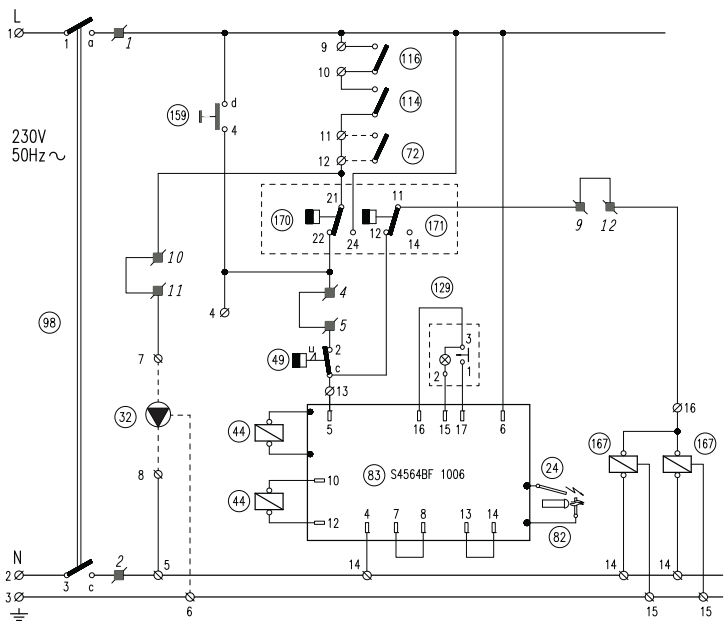
fig. 13 - Schema elettrico di principio mod. 119 - 136
