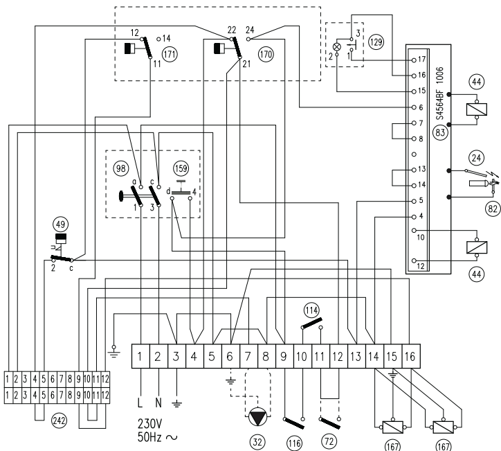
fig. 12 - Schema elettrico di allacciamento mod. 119 - 136
