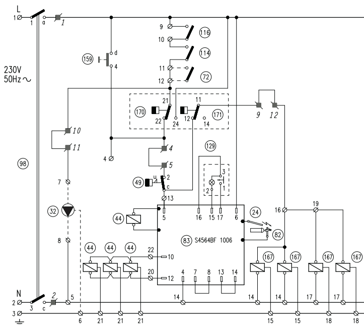
fig. 15 - Esquema eléctrico general mod. 153 ÷ 289
