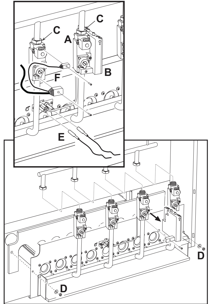
fig. 7 - Démontage et nettoyage des brûleurs
