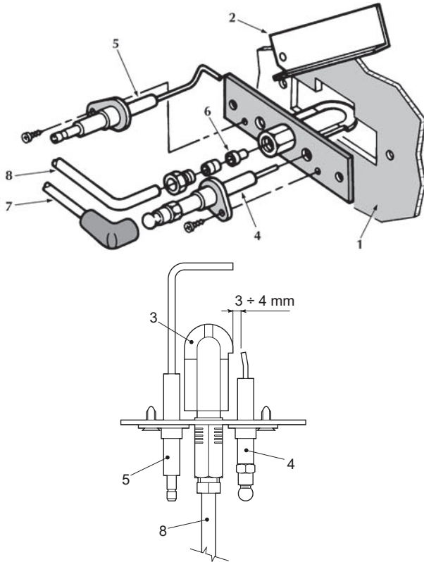
fig. 8 - Quemador piloto
