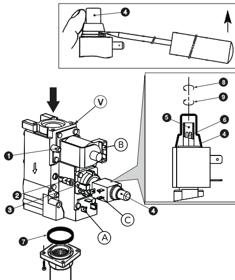
fig. 4 - Cambio de gas
