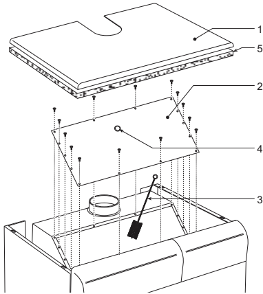
şek. 9 - Kombinin temizlenmesi
