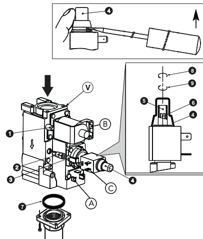
мал. 4 - Переведення на інший газ живлення
