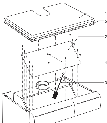
fig. 9 - Nettoyage de la chaudière
