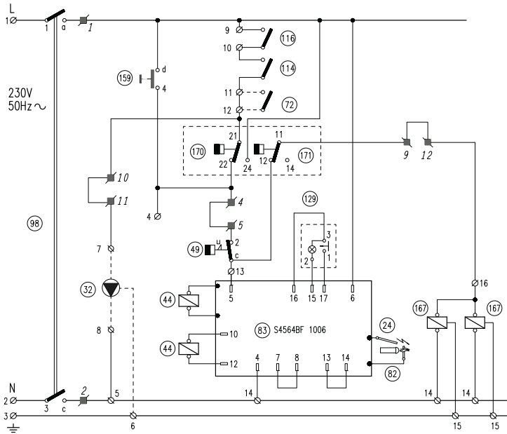
мал. 13 - Принципова електрична схема мод. 119 - 136
