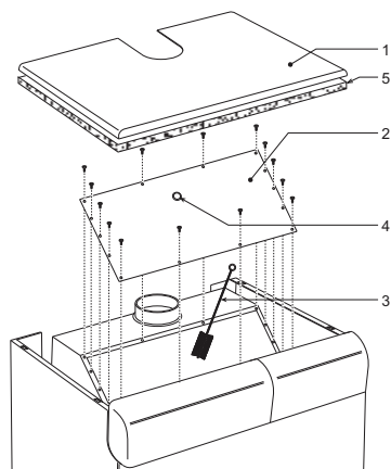
fig. 9 - Pulizia della caldaia
