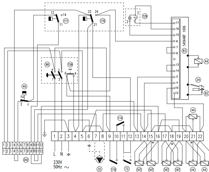
fig. 14 - Schema elettrico di allacciamento mod. 153 ÷ 289
