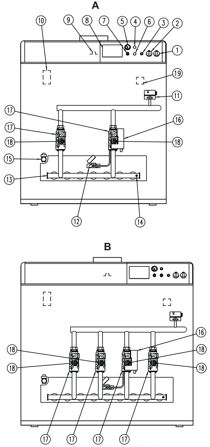
şek. 11 - Genel görünüm ve ana bileşenler
