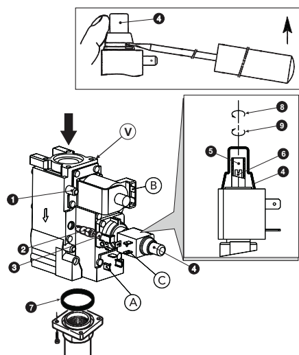
fig. 4 - Transformation du gaz d'alimentation
